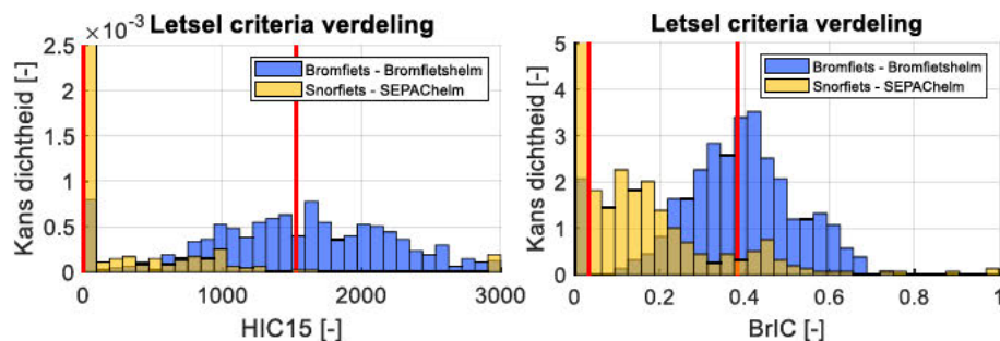
Figuur 25 Verdeling van de HIC15 (links) en BrIC (rechts) letselcriteria voor de bromfiets met volledig beschermende bromfietshelm en snorfiets met SEPAC-helm, in simulatiescenario 1. Rode lijn geeft 50% aan (mediaan).
